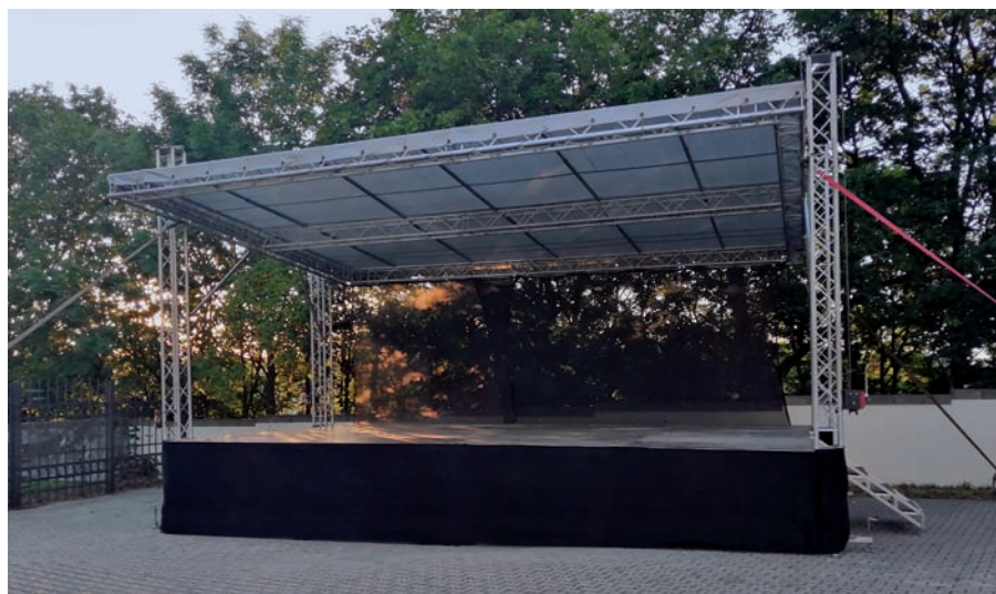
Pultová střecha 8 x 6 m Quatro
